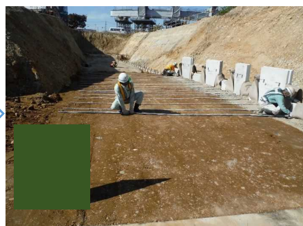
補強材設置
