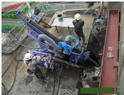
削孔
