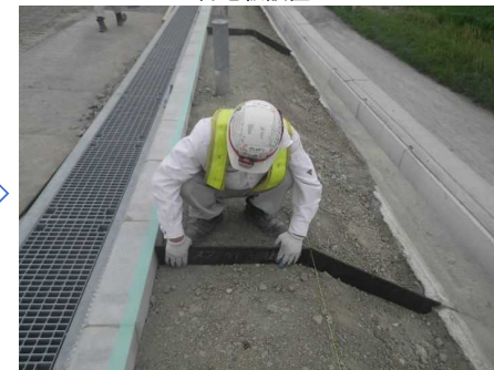
目地板設置
