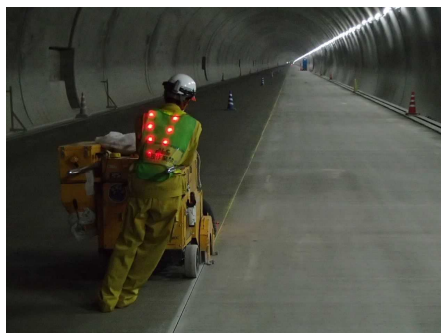
目地部切削
