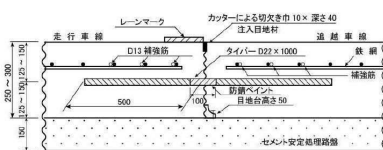
図－横断面図
