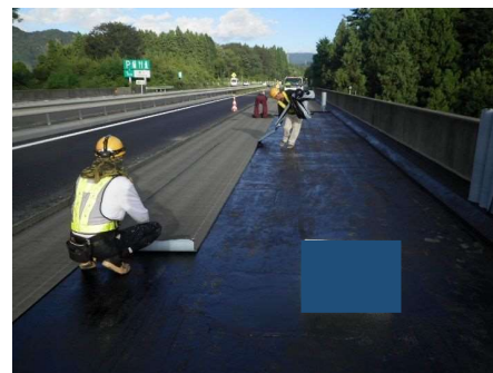
防水材施工
