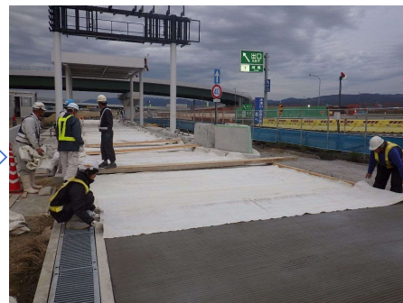
養生
