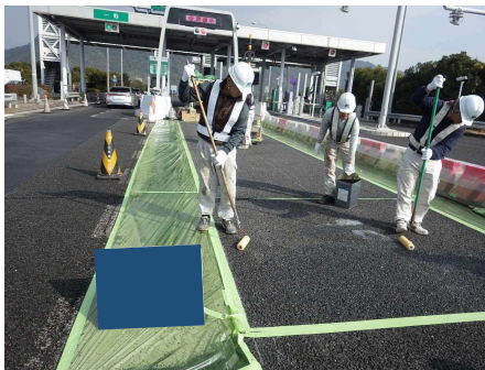
プライマー塗布
