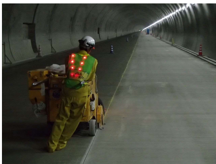
目地部切削
