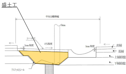
図-中央分離帯部
