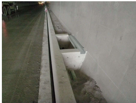
脱型枠後
