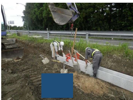
プレキャスト製品(U字溝)の据付
