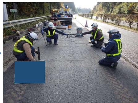
ループコイル埋設
