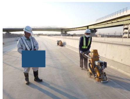
下地処理
