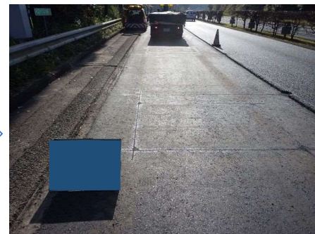
設置完了
