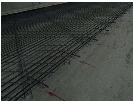
タイバー設置
