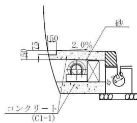
図－監査廊
