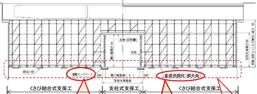
支保工基礎の施工例
