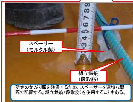
スペーサー配置
