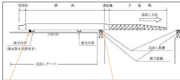
送出し装置による送出し
