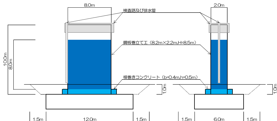
数量算出用の構造図
