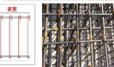
底版施工例
