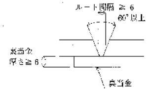
現場継ぎ形状
