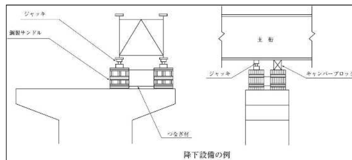
降下設備（サンドル降下）概念図
