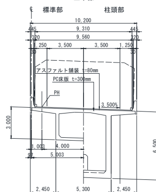
単一断面 上り線
