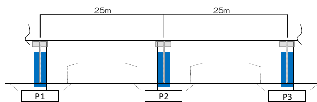
橋脚配置図
