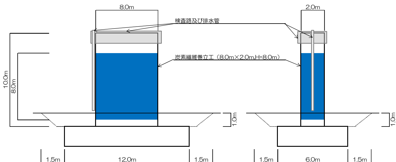
形状図
