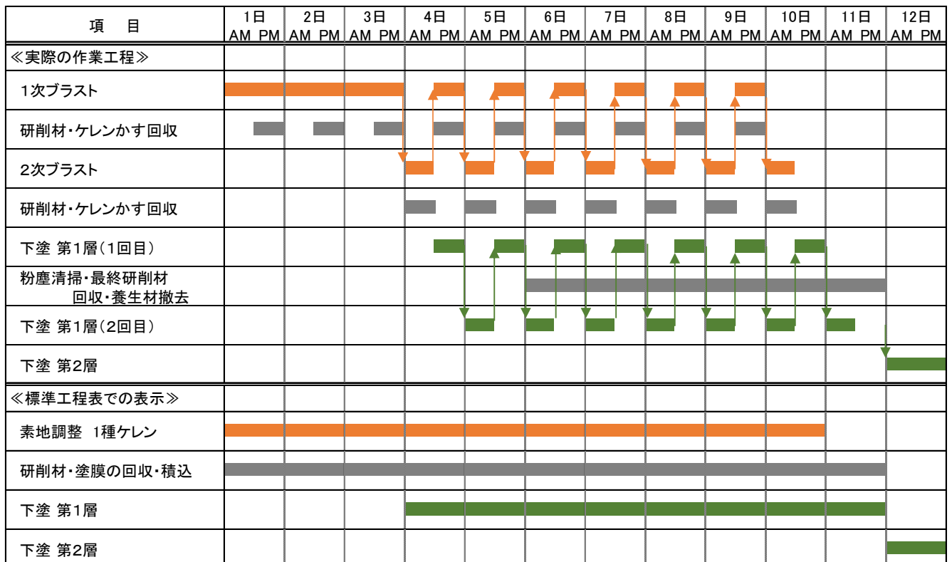
図 5-14-2 塗装面積 500 m 2 あたりのブラスト～塗装作業までの施工工程（概念図）
