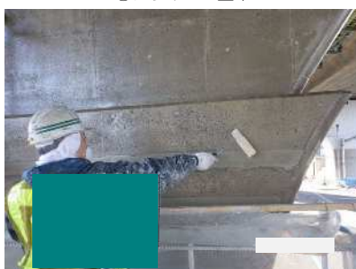
②プライマー塗布
