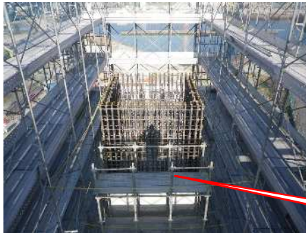
横梁用支保工（支柱式）
