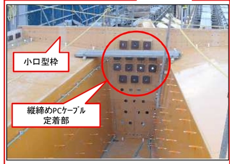
施工継目 小口型枠（縦締めPCケーブル定着部）
