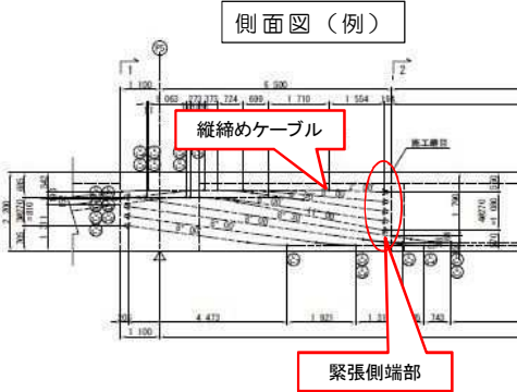
縦 締 め 緊 張 状 況
