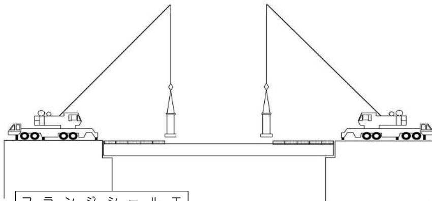
フランジシール工
