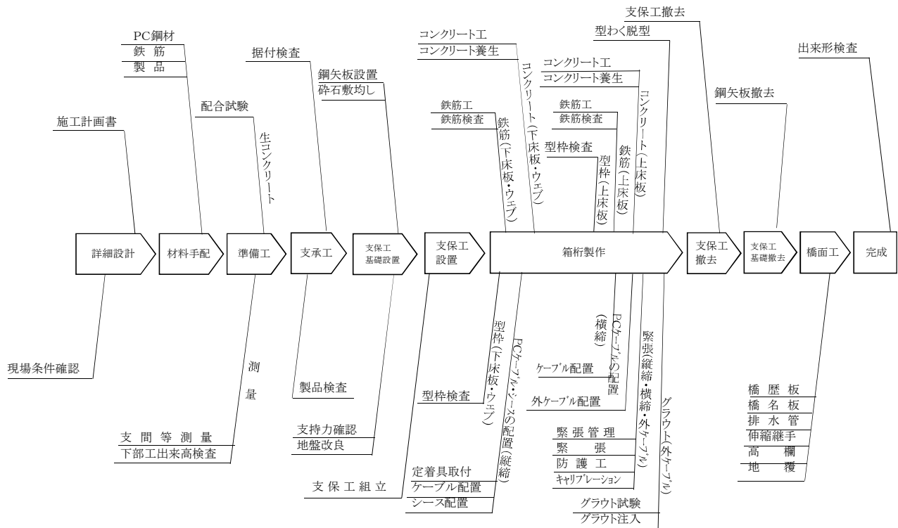
PC箱桁橋(場所打ち)工事施工の流れ
