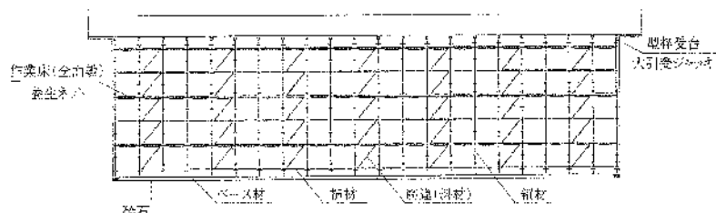
くさび結合式支保工
