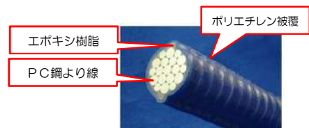
プレグラウトPCケーブル
