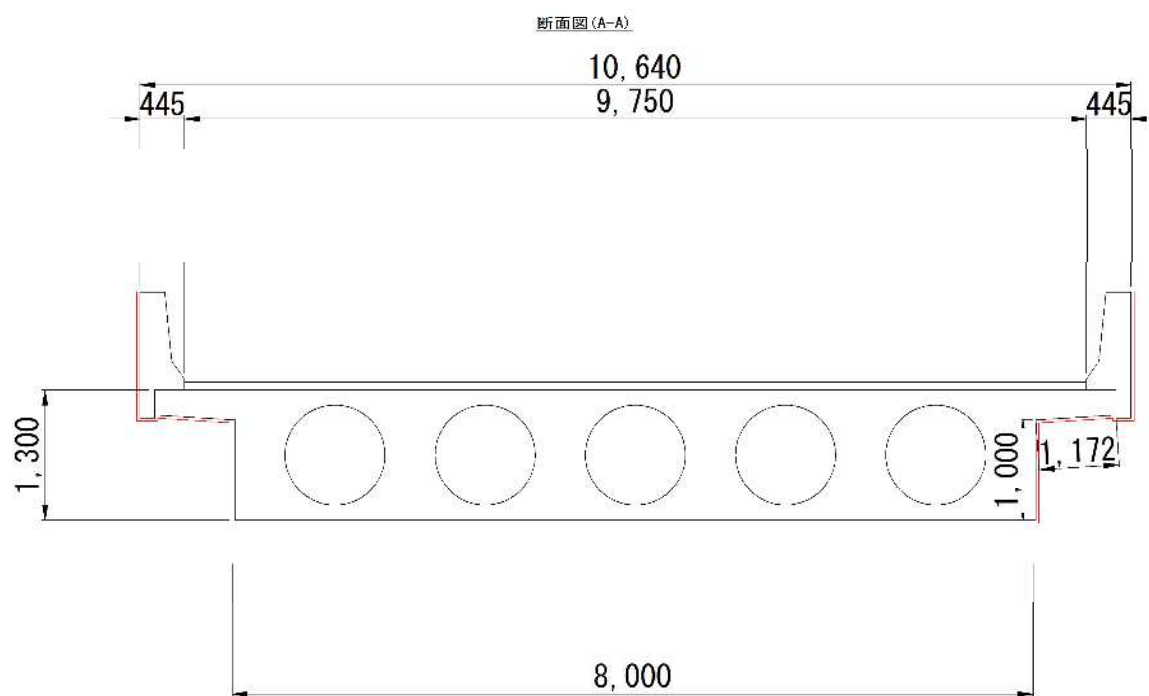
数量算出用の構造図
