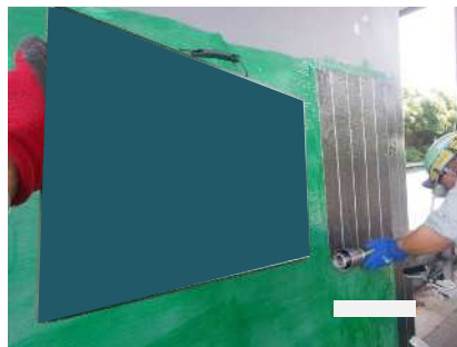
炭素繊維シート貼付け
