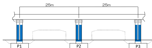
橋脚配置図
