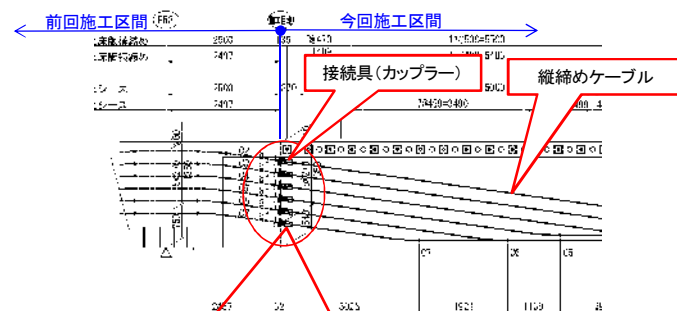
接 続 箇 所 側 面 図 ( 例 )
