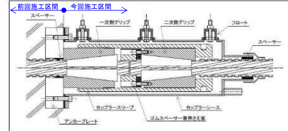
■ 接続およびカップラーシース取り付け後の状況
