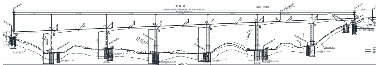
単一断面 上り線
