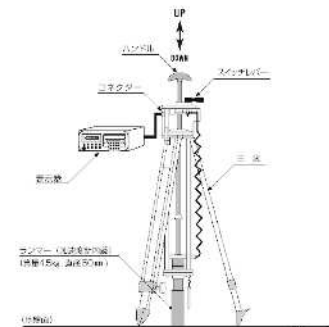
簡易支持力測定器(キャスボル)
