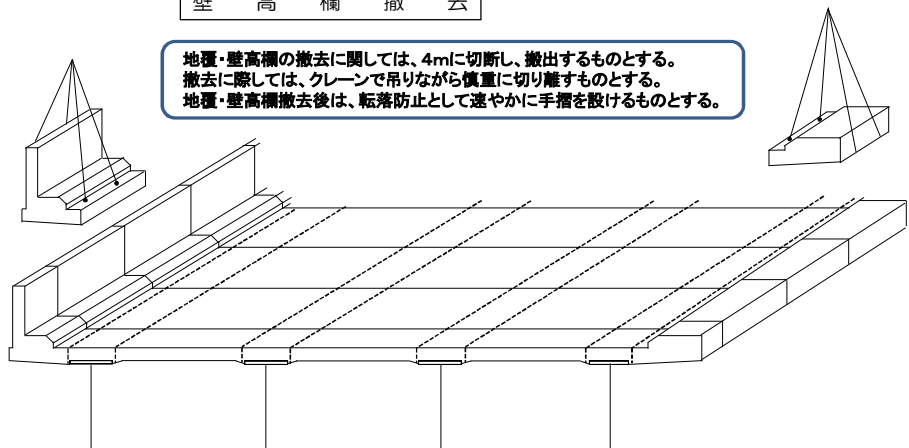
壁高欄撤去
