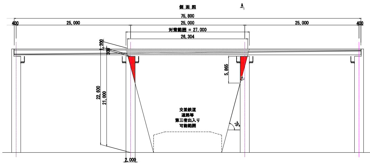
数量算出用の構造図
