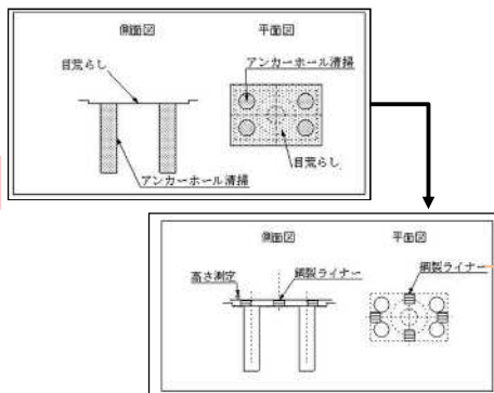
支承据付
