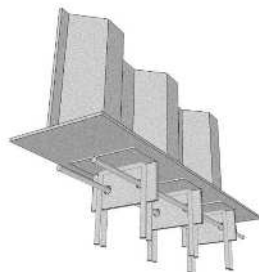
a) アングルジベル接合
