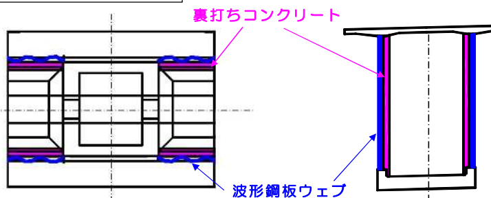
裏打ちコンクリート
