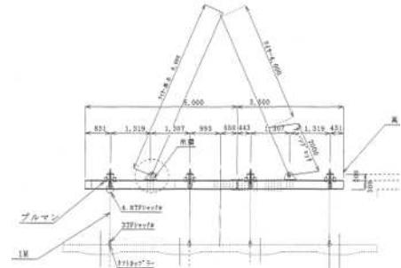
新設床版吊り治具
