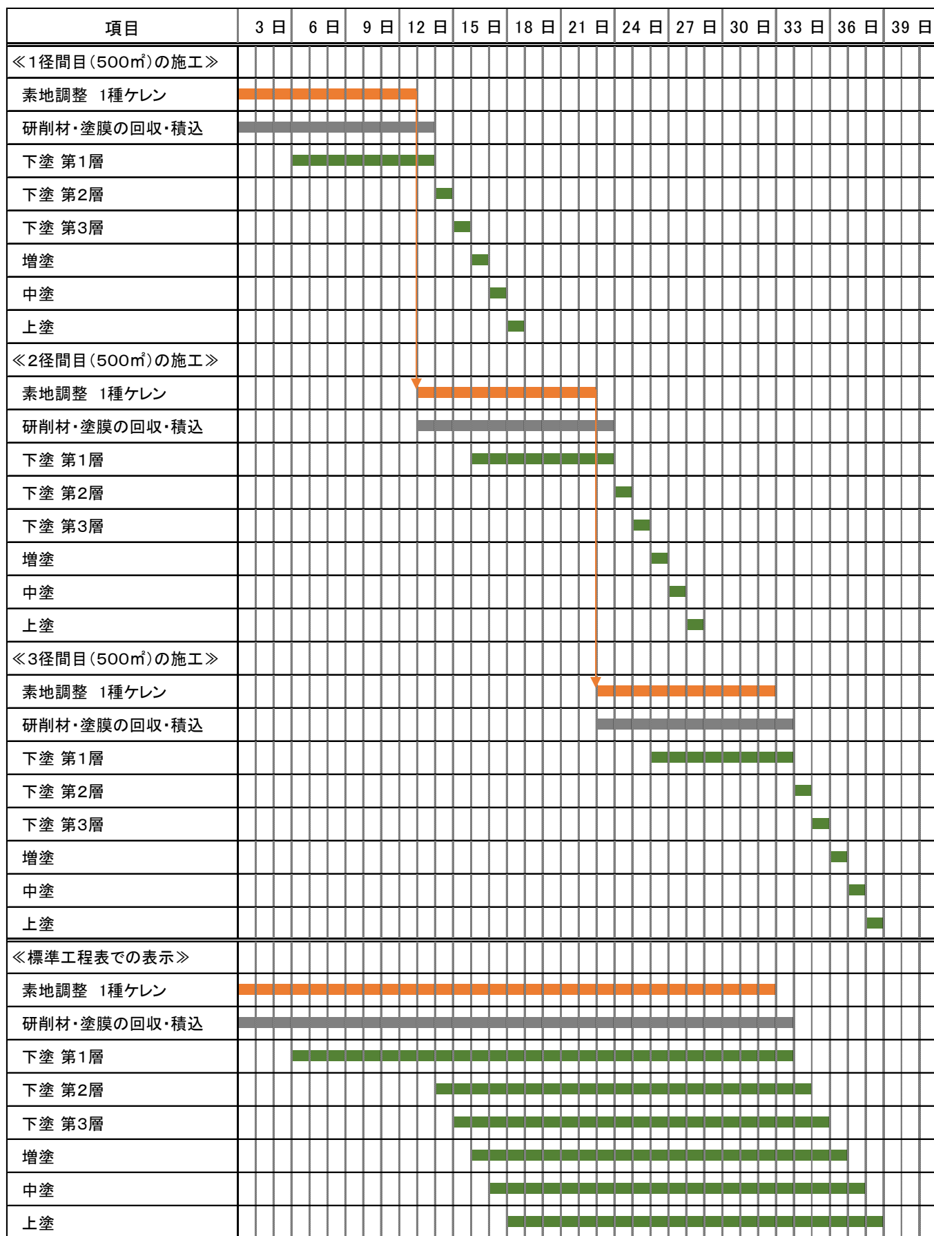
図 5-14-3 複数径間の場合のブラスト～塗装作業までの施工工程（概念図）
