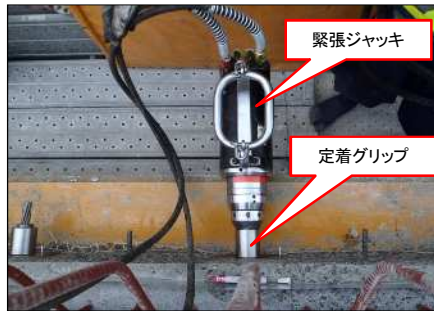
横 締 め 緊 張 状 況
