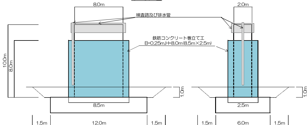
形状図
