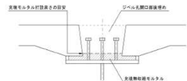
無収縮モルタルの打設高
