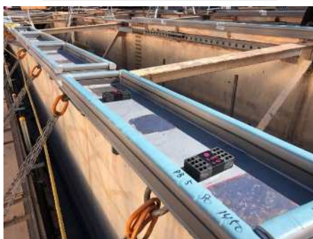
フランジシール工
