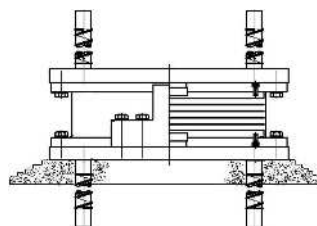
ゴム支承の模式図
