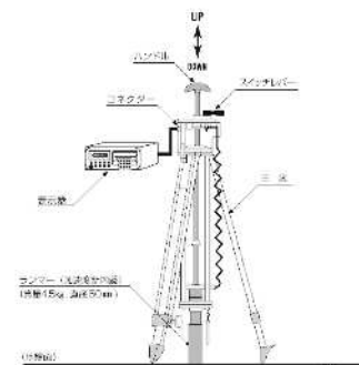
簡易支持力測定器(キャスホル)
