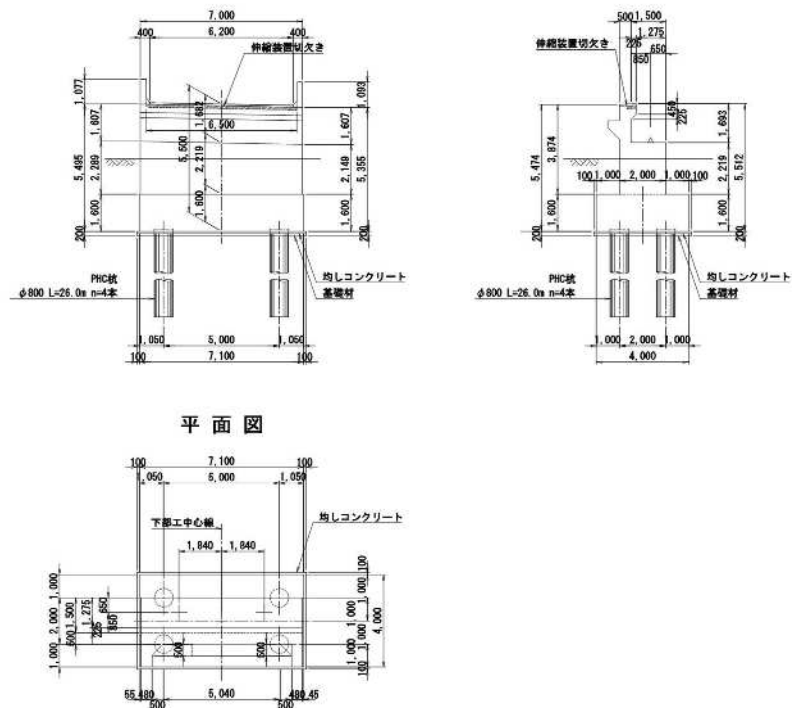
側面図
