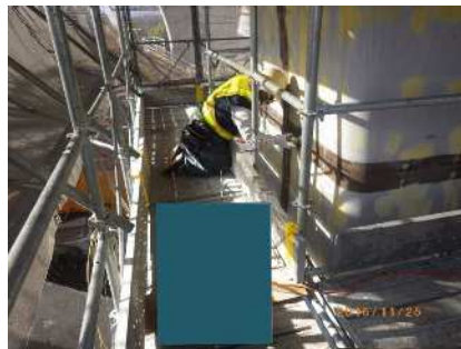
溶接部ケレン状況
