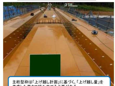
型枠組立
