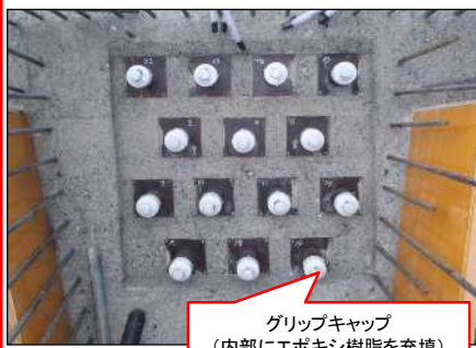
縦 締 め 後 処 理 完 了
