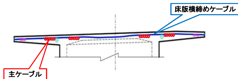
主ケーブル・床版横締めケーブル
