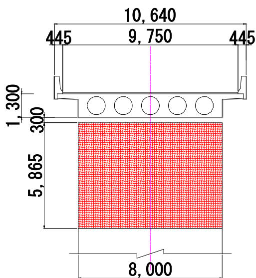
断面図 (A-A)
