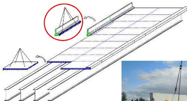
壁高欄撤去
