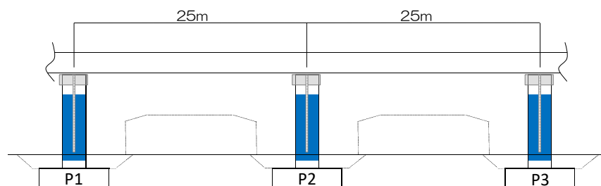
橋脚配置図
