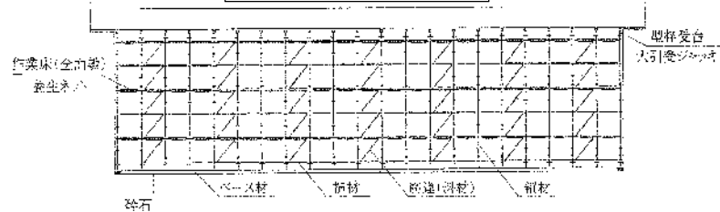
くさび結合式支保工施工例
