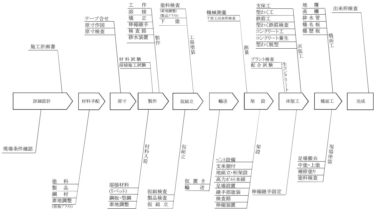
鋼橋(桁橋)工事施工の流れ(トラッククレーンベント工法)
