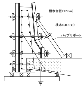
壁高欄型枠組立状況
