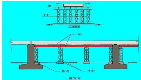
支柱式支保工（H鋼梁）
