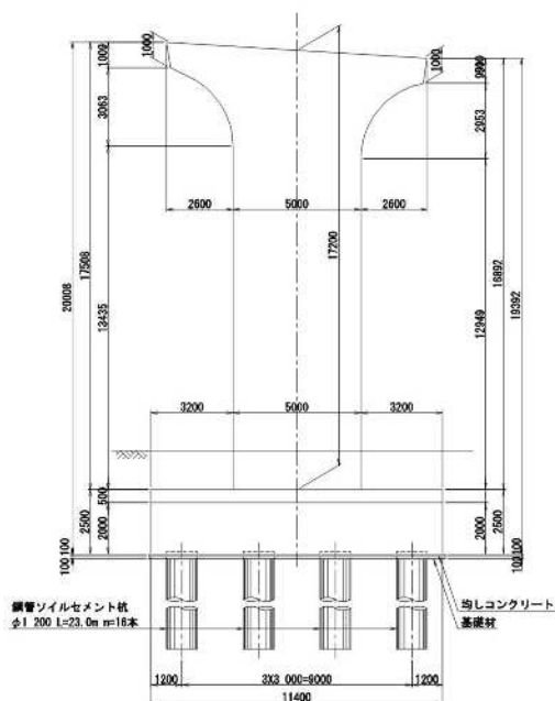
断面図
