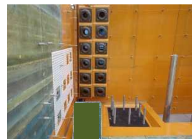
緊張端付近の型枠状況
