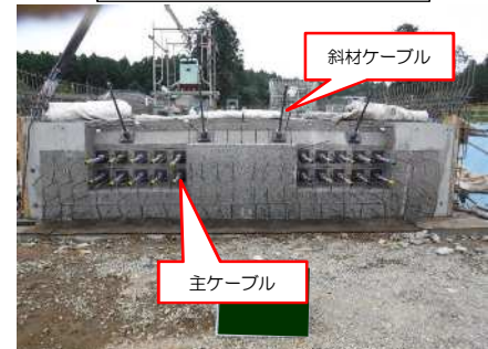
定着具セット
