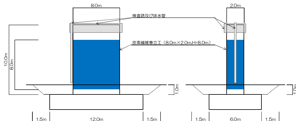
数量算出用の構造図
