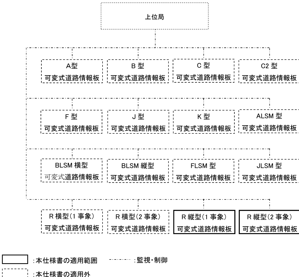
図1-2-1 全体構成
